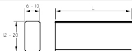
TERMINACIÓN PARA PÉRGOLA 20x10
