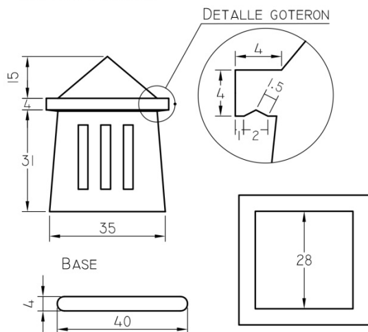
CHIMENEA 35x35
